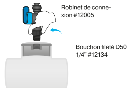
Raccord en T
