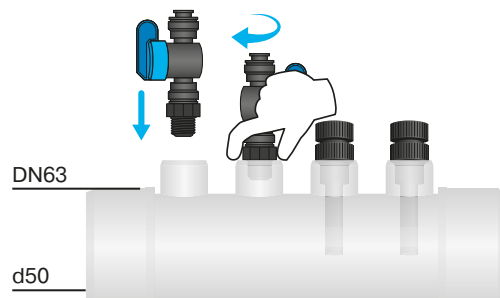
Collecteur d'injection d50/DN63 4x 1/4" #13395
