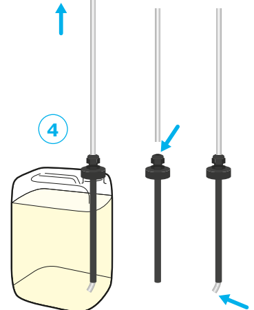
Sací sada pro 20l kanystr #13415
