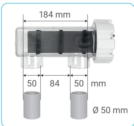
Elektroda TE-25
