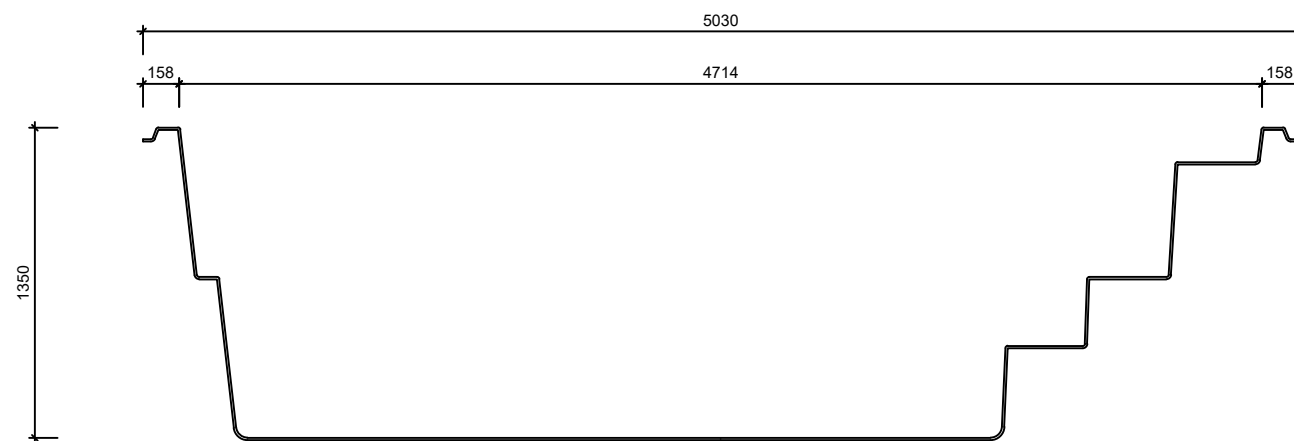
Schnitt A-A
