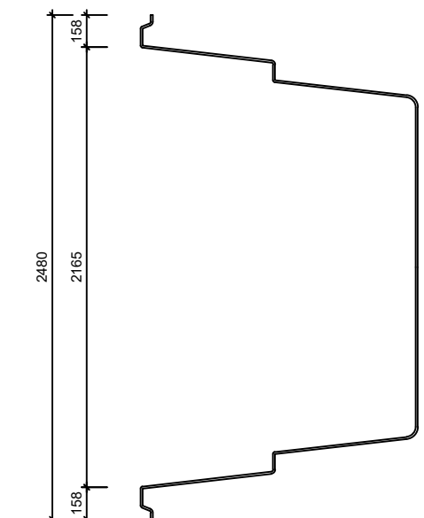
Schnitt B-B
