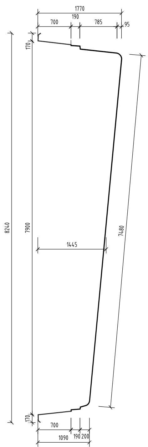
COUPE 2 - 2 M 1:50
