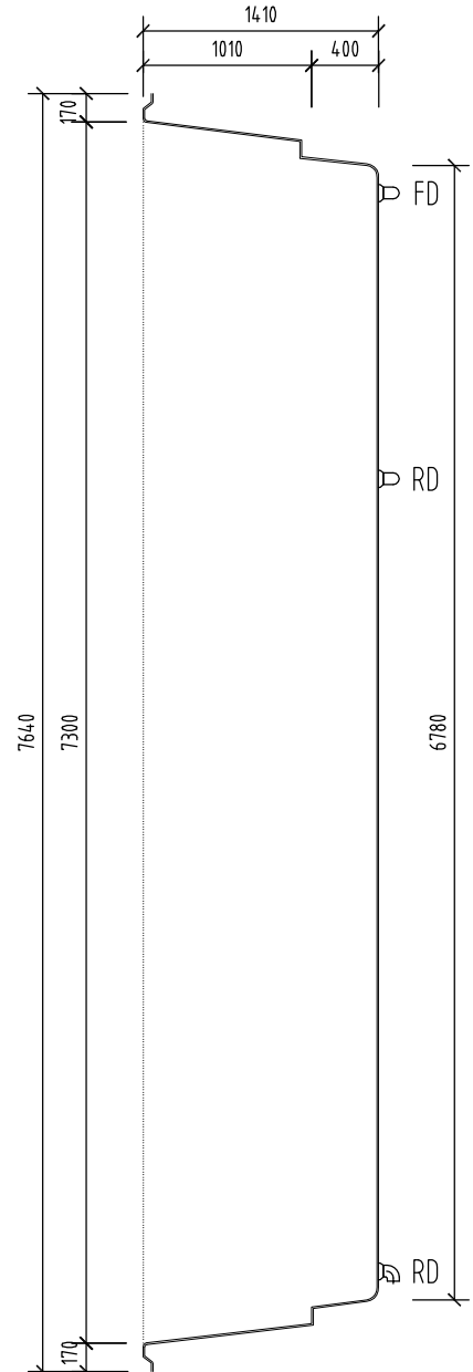
REZ 2-2 M 1:50 LONGITUDINAL SECTION QUERSCHNITT
