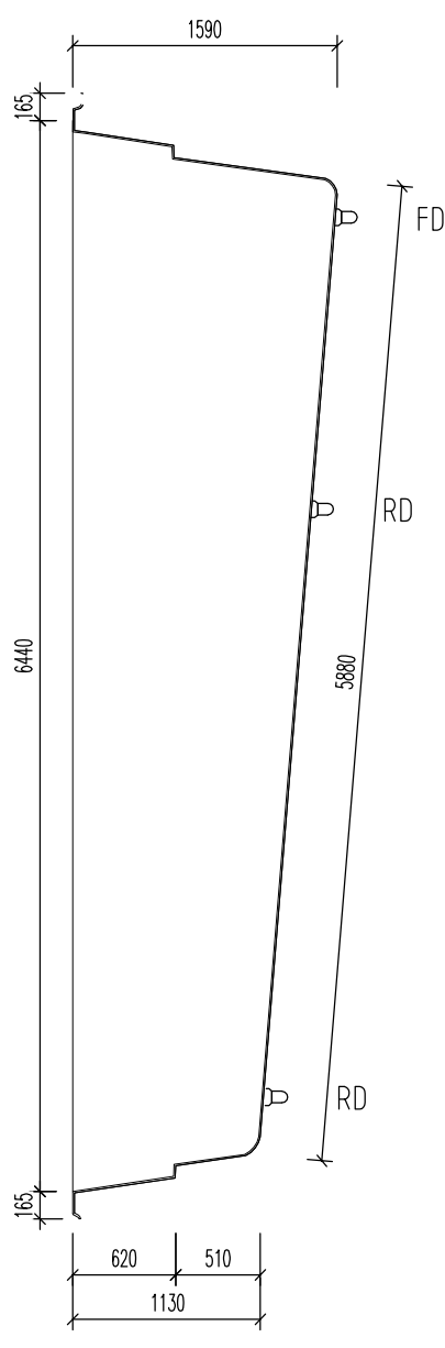
COUPE 2 - 2 M 1:50
