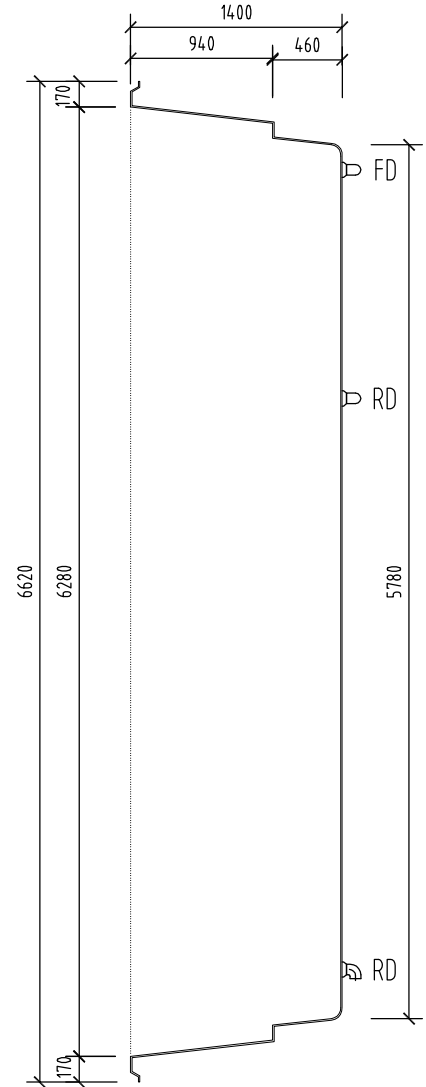
REZ 2 - 2 M 1:50 LONGITUDINAL SECTION QUERSCHNITT
