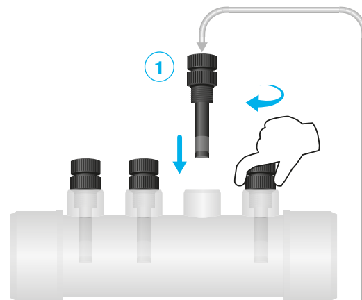
Impfstrecke 4x 1/4" # 13395
